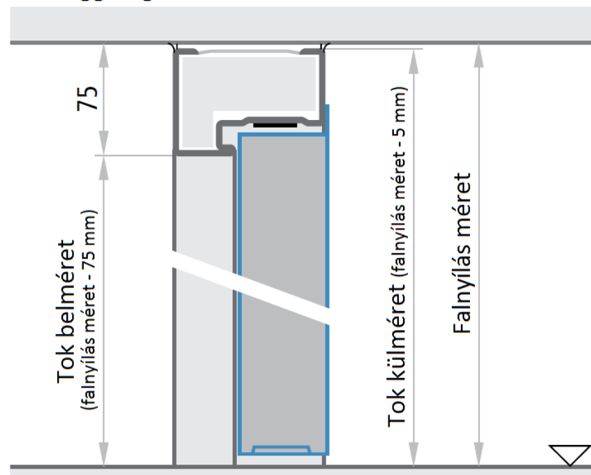
Függőleges metszet
