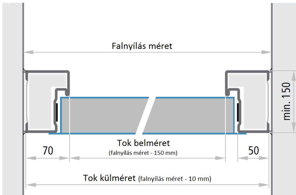
Vízszintes metszet
